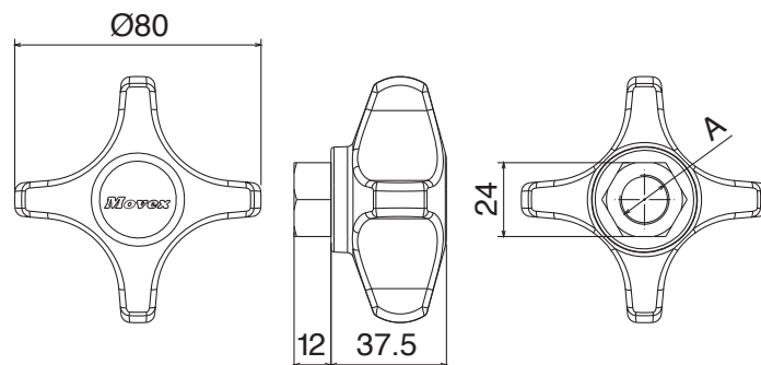
Volantino Ø80 / Star knob Ø80 / Sterngriff Ø80
