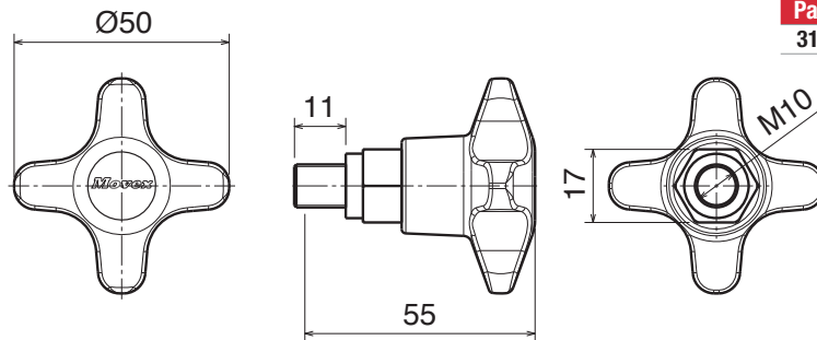
Volantino / Star knob / Sterngriff
