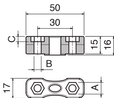
Bloccetto giunzione / Connecting element / Verbindungselement
