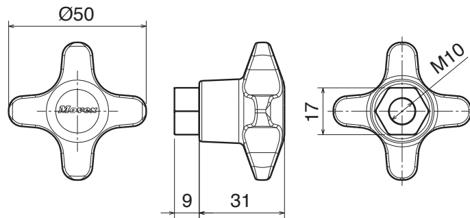
Volantino / Star knob / Sterngriff
