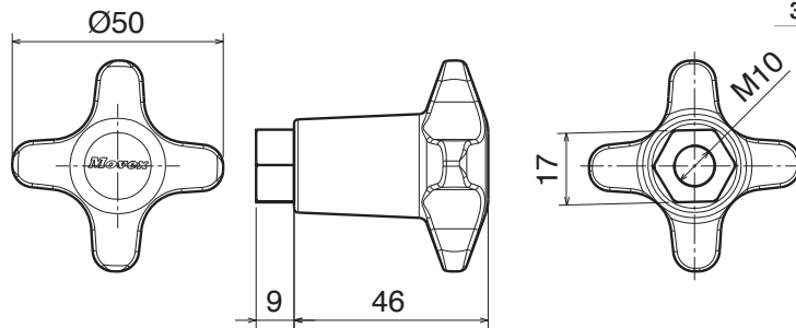
Volantino / Star knob / Sterngriff
